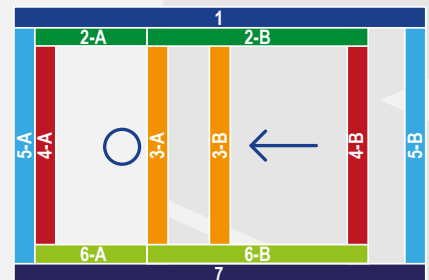
DESPIECE PERFILES VENTANA CORREDIZA 8025 (MARCO CON DOS NAVES UNA FIJA Y UNA CORREDIZA)
