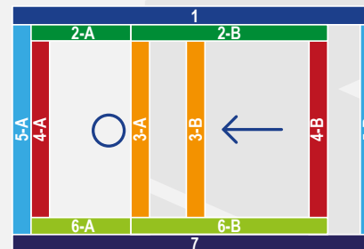
DESPIECE PERFILES VENTANA CORREDIZA 8025 (MARCO CON DOS NAVES UNA FIJA Y UNA CORREDIZA)
